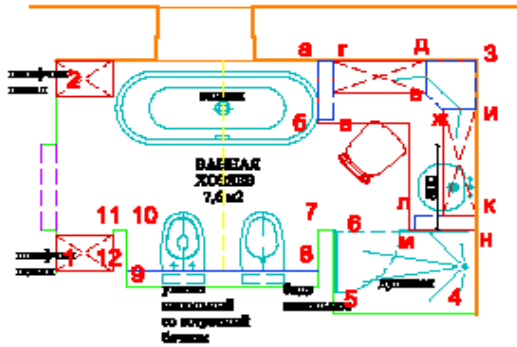
ВАННАЯ ХОЗЯИН на 2-ом ЭТАЖЕ (фронталь: план расположения мебели и сантехники)
